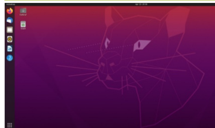
Linux
